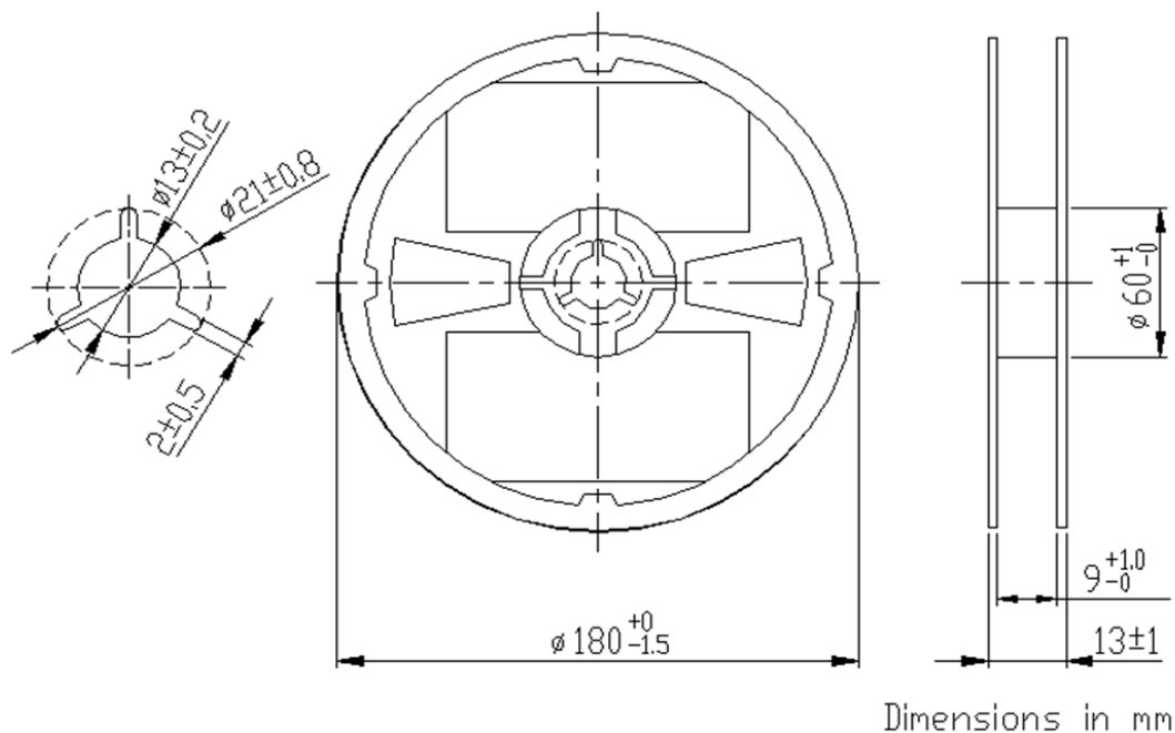
Reel Dimensions
